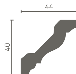
DD21 — 40x44x2000 мм
